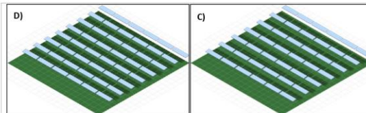
Figura 7. Distribuições espaciais das configurações através do software PVSyst para as densidades de módulos por hectare que proporcionam as taxas de ocupação do solo de A) 0,66 (SF-Ref. 0,66); B) de 0,39 (SAF-0,39); C) de 0,33 (SAF-0,33); e D) de 0,28 (SAF-0,28). Obs. SF-Ref é o Sistema fotovoltaico de referência, isto é, com a densidade de módulos utilizada em uma usina fotovoltaica convencional.
