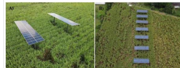
Figura 2. Vista aérea do sistema agrofotovoltaico instalado em Rio Largo – AL.
