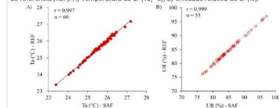
Figura 3: Comparação entre variáveis atmosféricas no sistema agrofotovoltaico (SAF) e cultivo de referência (REF): A) Temperatura do ar (Ta, °C); B) Umidade relativa do ar (%).
