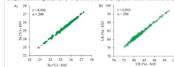
Figura 4: Comparação entre variáveis atmosféricas no sistema agrofotovoltaico (SAF) e na estação meteorológica (EM): A) Temperatura do ar (Ta, °C); B) Umidade relativa do ar (%).
