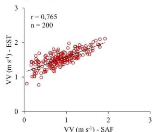
Figura 6: Comparação entre a velocidade do vento (VV, m s -1 ) no sistema agrofotovoltaico (SAF) e na estação meteorológica (EM).
