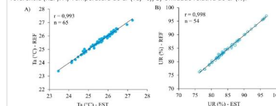
Figura 5: Comparação entre variáveis atmosféricas na estação meteorológica (EM) e cultivo de referência (REF): A) Temperatura do ar (Ta, °C); B) Umidade relativa do ar (%).
